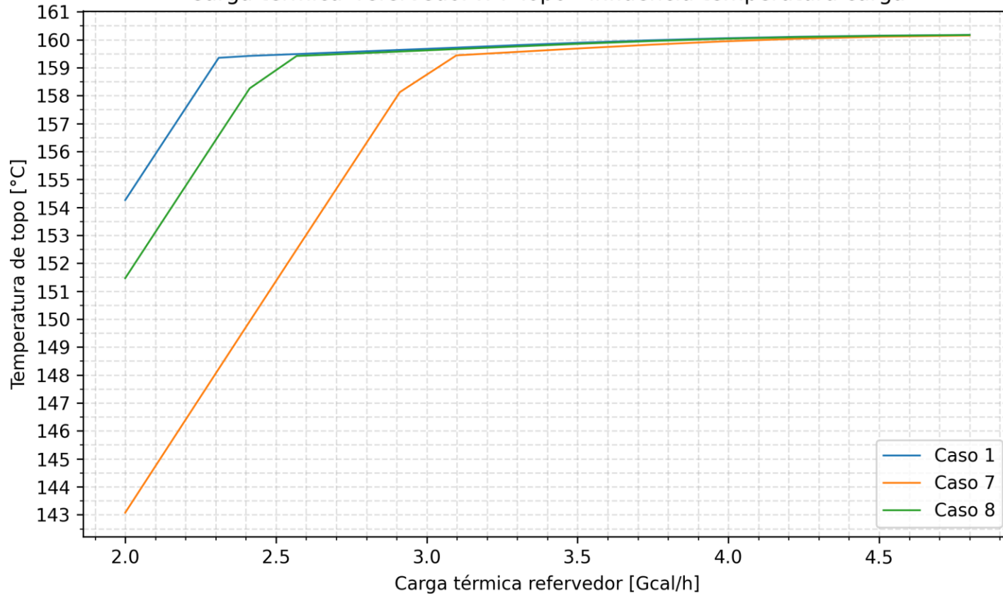
Carga térmica refeedor x T Topo - influência temperatura carga
